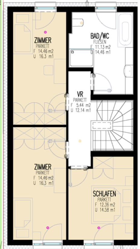
1. OBERGESCHOSS
