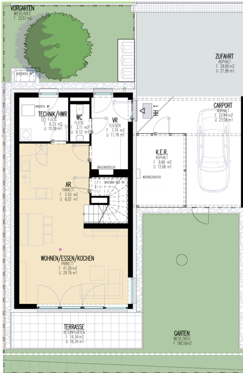
ERDGESCHOSS
